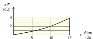
- Variación de la Figura de Ruido F con la atenuación introducida
